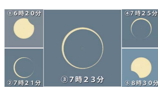
【図】5月21日金環日食の経過(ステラナビゲータで作成)
