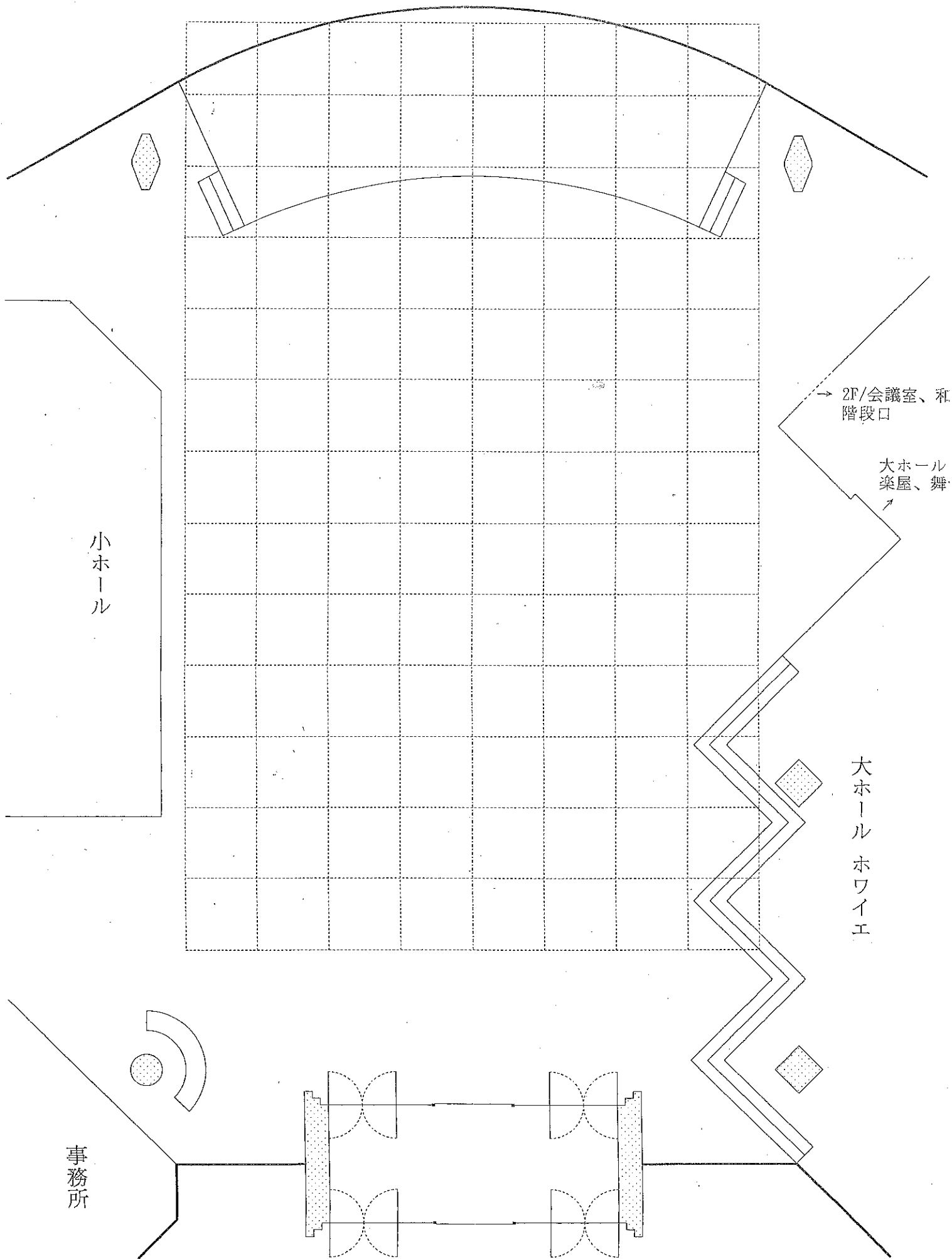
小林市文化会館 エントランス平面図 縮尺/1:100
