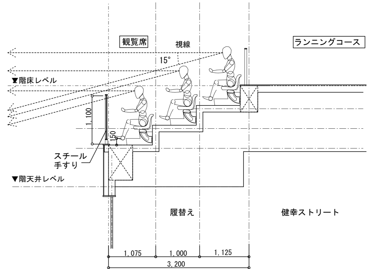
断面図 S=50
