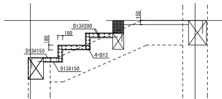
S11 配筋詳細図
